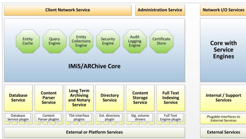
Slika 1: Shematični prikaz arhitekture strežniške komponente IMiS®/ARChive Server
