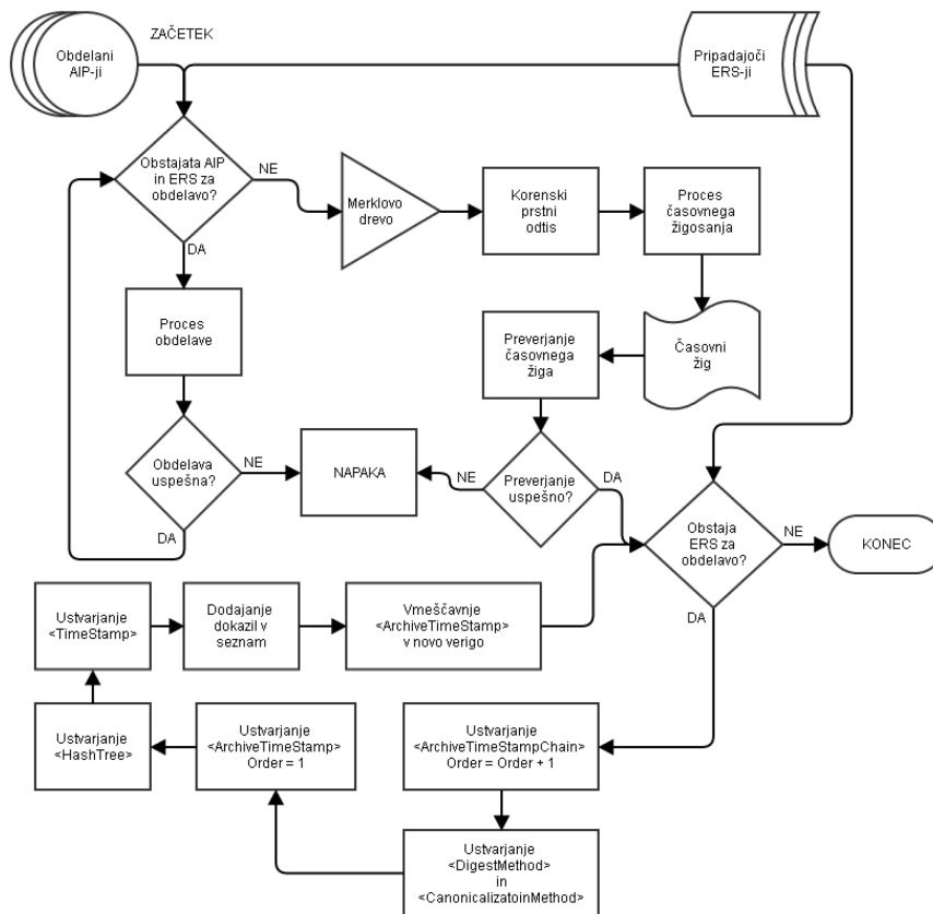
Slika 23: Postopek kompleksnega podaljševanja z Merklvim drevesom
