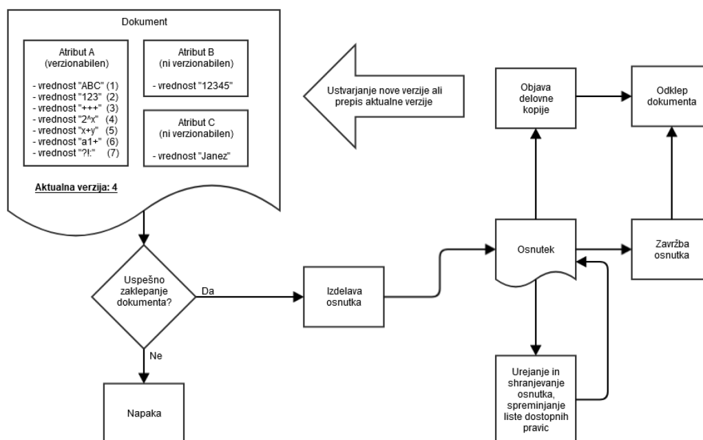
Slika 34: Proces verzioniranja
