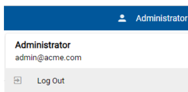
Slika 61: Odjava uporabnika
