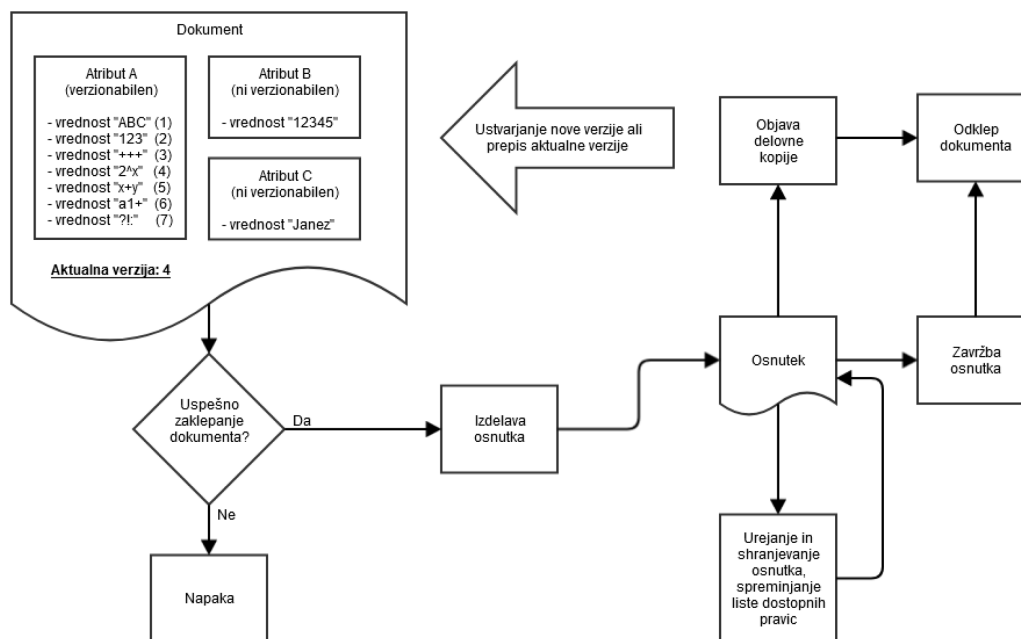
Slika 35: Proces verzioniranja
