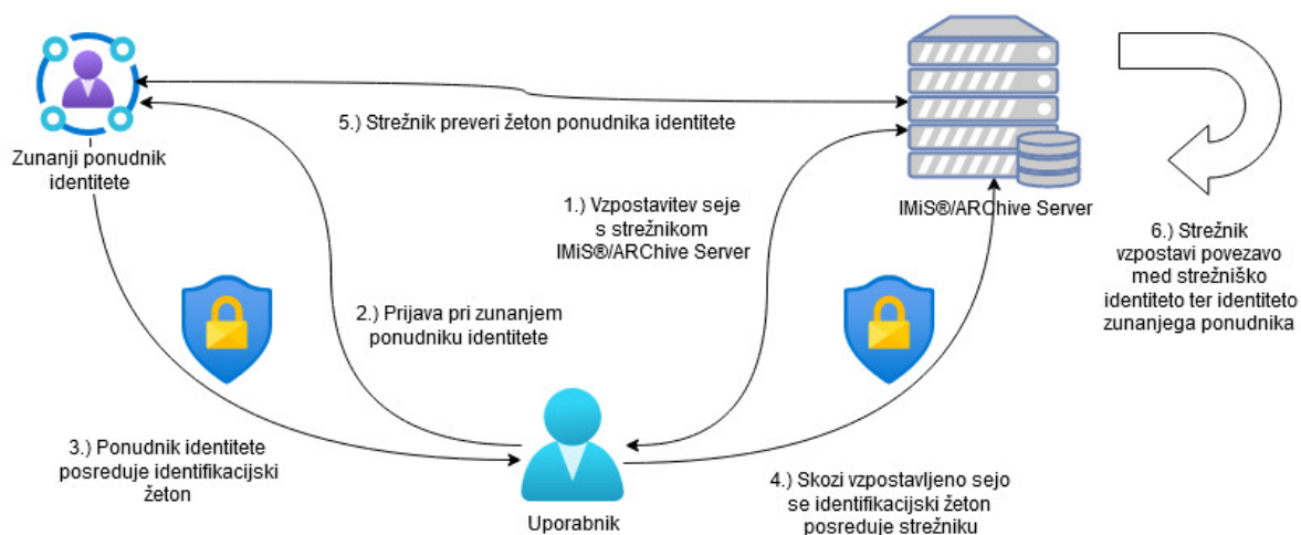
Slika 32: Povezovanje identitet
