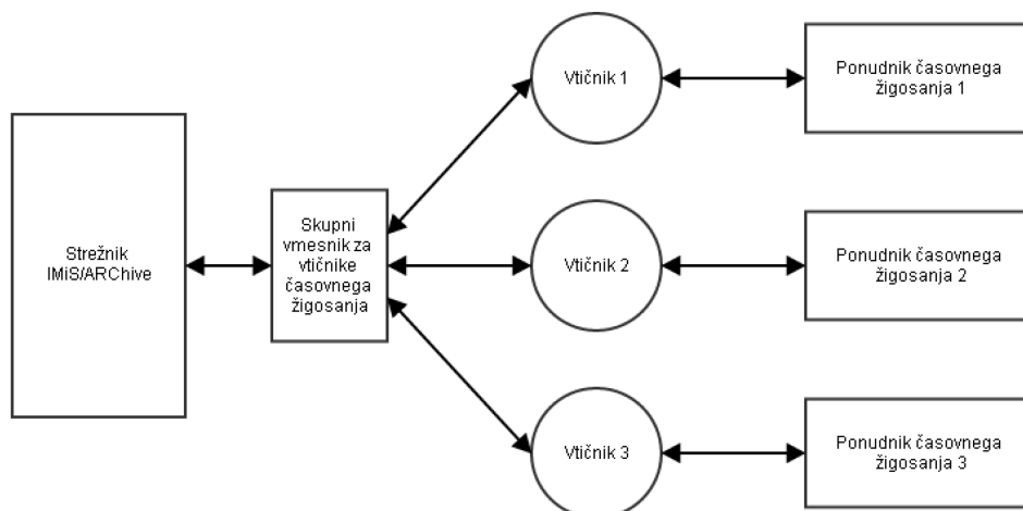
Slika 24: Koncept vtičnikov
